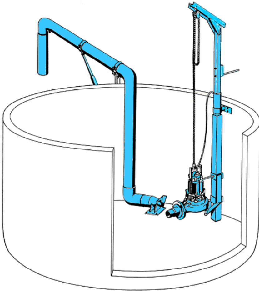
F-PUMPPU ASENNETTUNA YHDISTETTYYN KIERRÄTYS JA ETEENPÄIN PUMPPAUS JÄRJESTELMÄÄN
